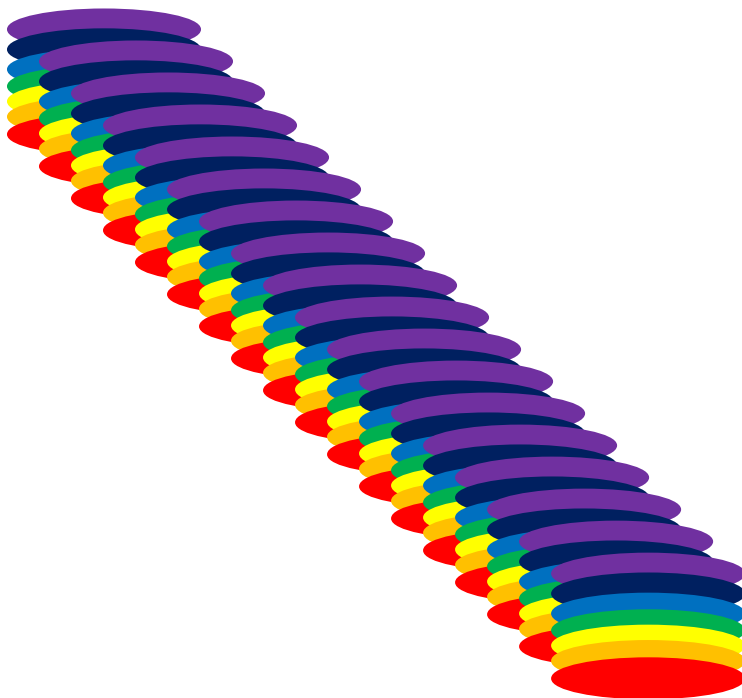
Figur 1: Kvanta av energi eller kvanta av mörk energi 10^{-29}\text{g}/\text{cm}^3 absorberas genom m partikel och bär kvanta av massa 3, e^{-61}\text{g} i 5\,474\,959\,764\,225\,000\text{ m}/\text{sekund} .
