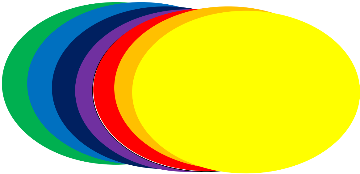
Figur 8: Hela vårt universum där månen, stjärnor, solar, planeter, galaxer, galaxhopar, supergalaxhopar, nebulosor, atomer, människor, djur, växter och allt liv har sina platser har 6 dubletter exakt som originalet i sex symmetriska universum.
