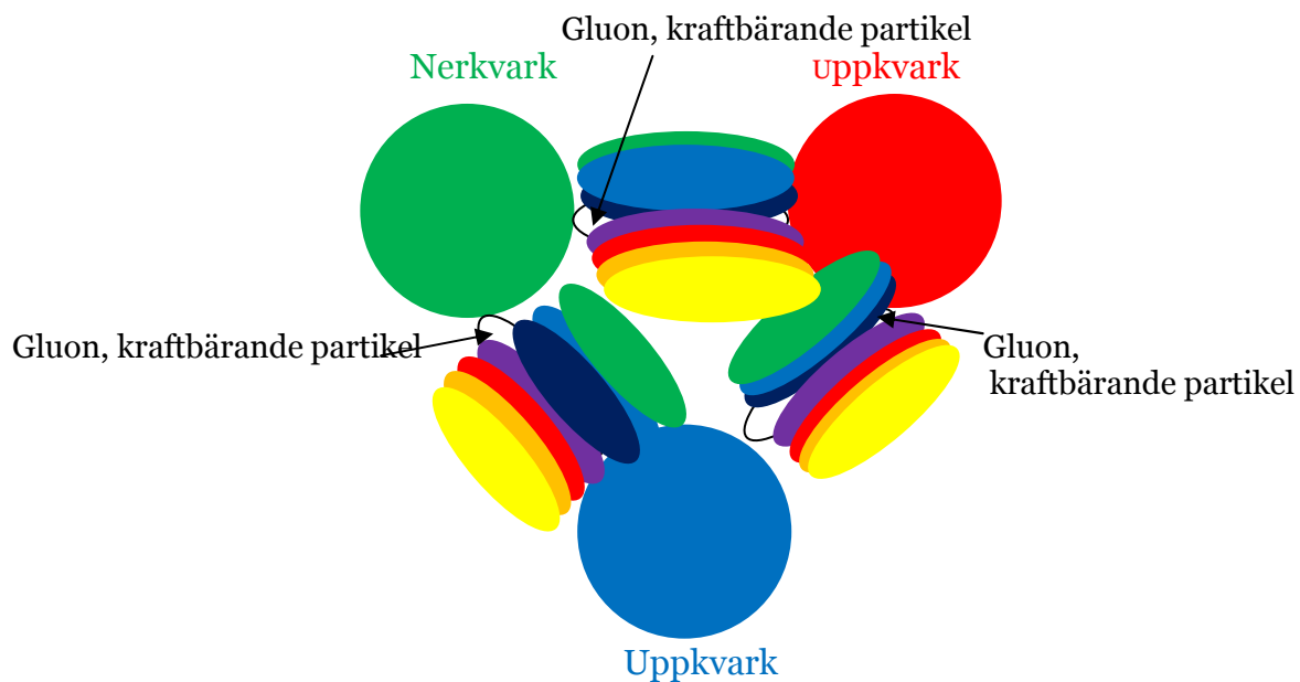
Figur 3: Kvarkarna i protonen och gluoner (kraftbärande partiklar) binder kvarkarna. Var och en av gluoner har 6 dubletter i de sex symmetriska universum.
