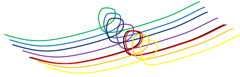
Figur 4: Ett hårstrå, vilket är ungefär 25 mikrometer tjock har 6 dubletter exakt som originalet i sex symmetriska universum.
