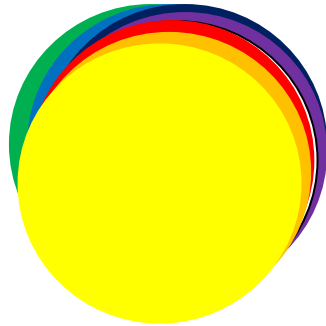
Figur 7: Jorden, där vi bor i miljoner år har 6 dubletter exakt som originalet i de sex symmetriska universum.
